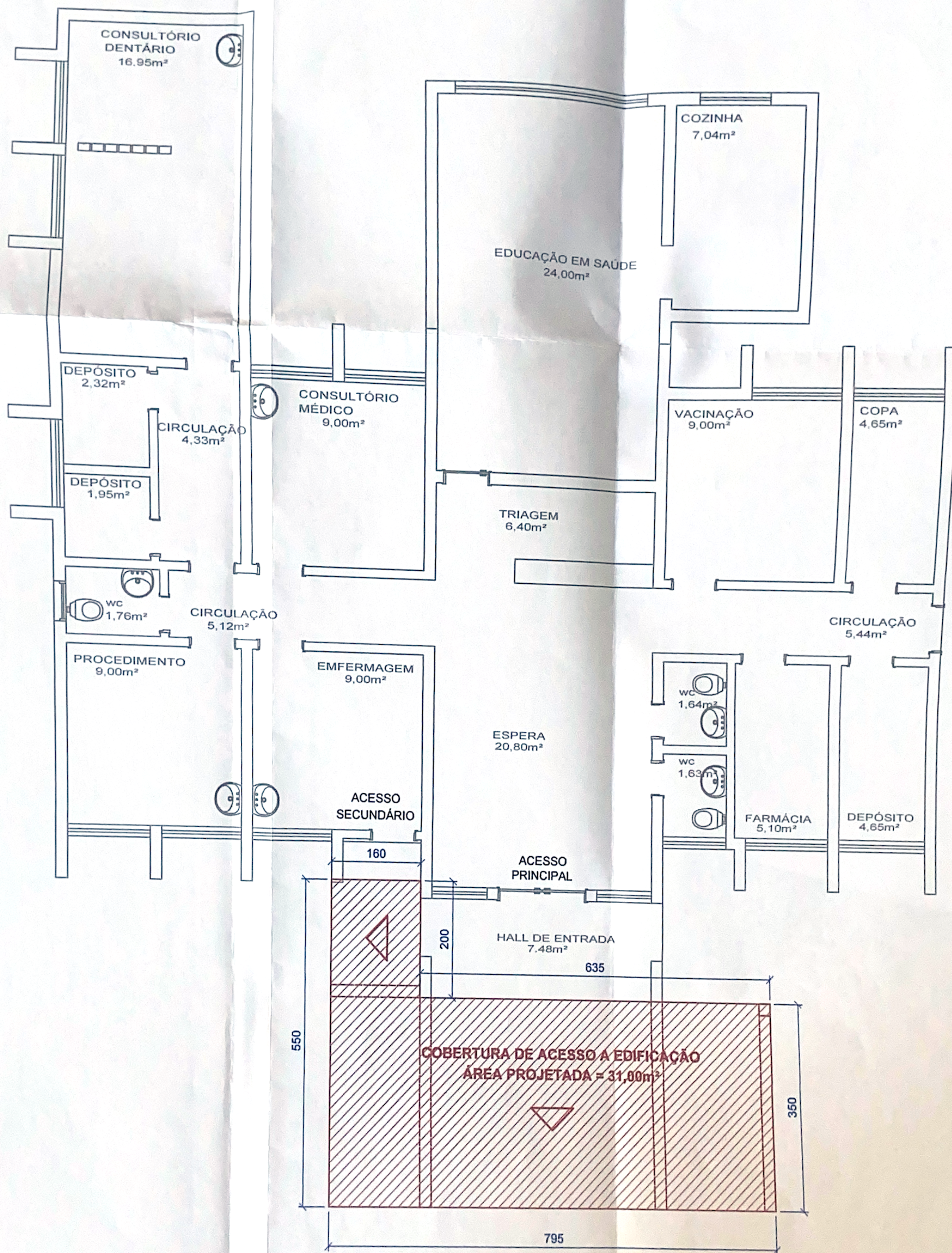
PLANTA DE IMPLANTAÇÃO ESCALA 1:75
